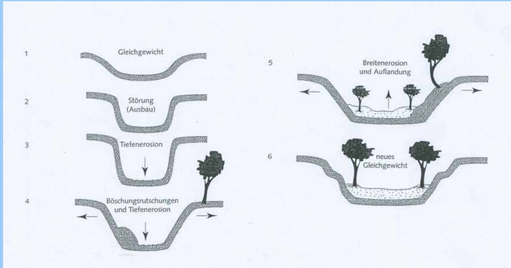
Entwicklungsphasen von Erosionsgewässern (nach Klaus KERN)
